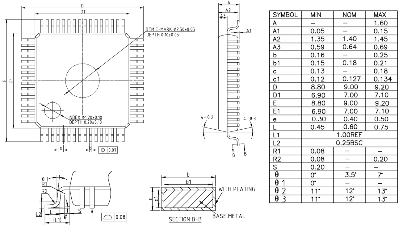
图 6-1 BR6210 封装尺寸图
