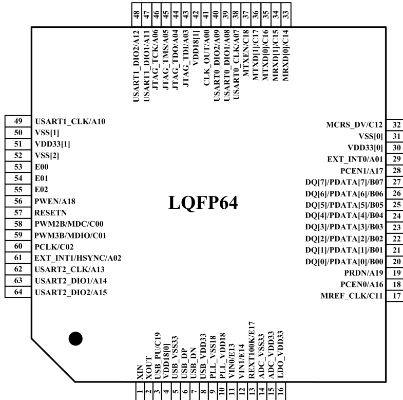
图 3-1 BR6210 引脚分布图
