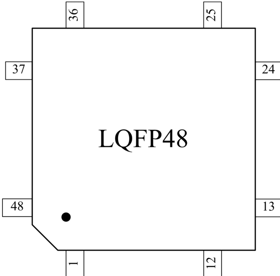
图 3-1 BR6211 封装形式
