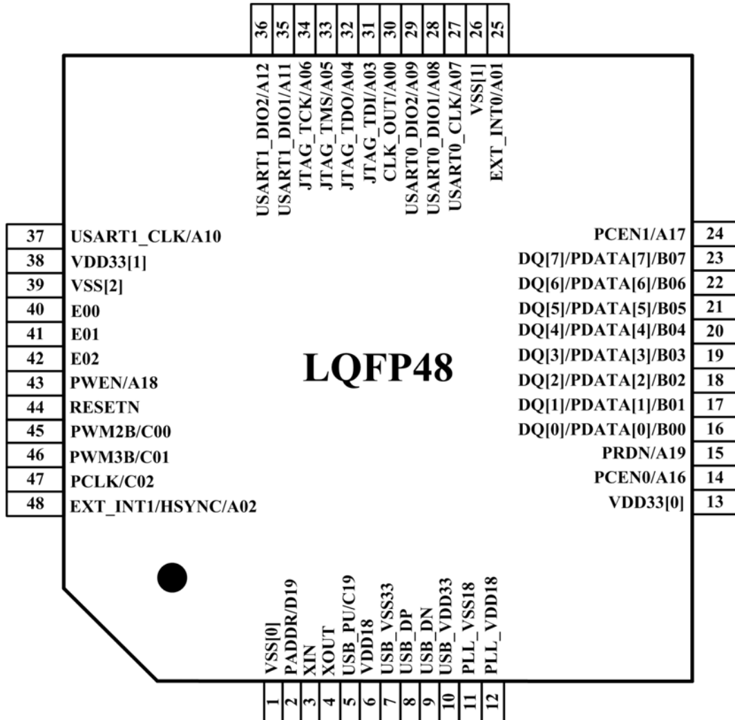
图 3-2 BR6211 引脚分布图
