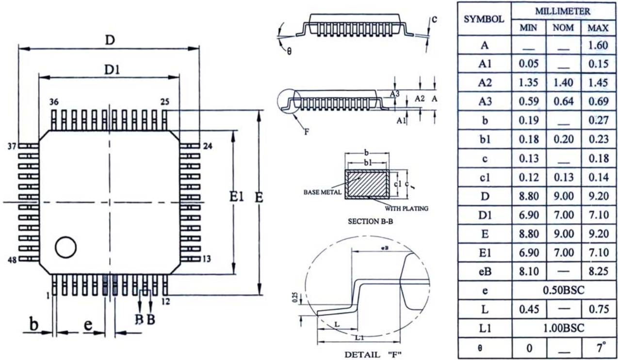
图 6-1 BR6211 机械结构
