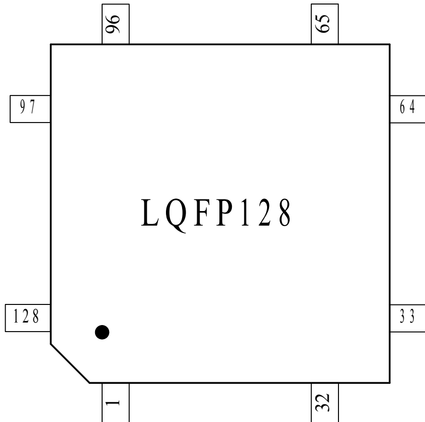
图 3-1 BR8220 封装形式
