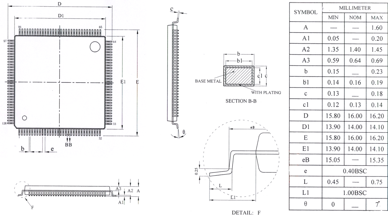
图 6-1 BR8220 封装尺寸图
