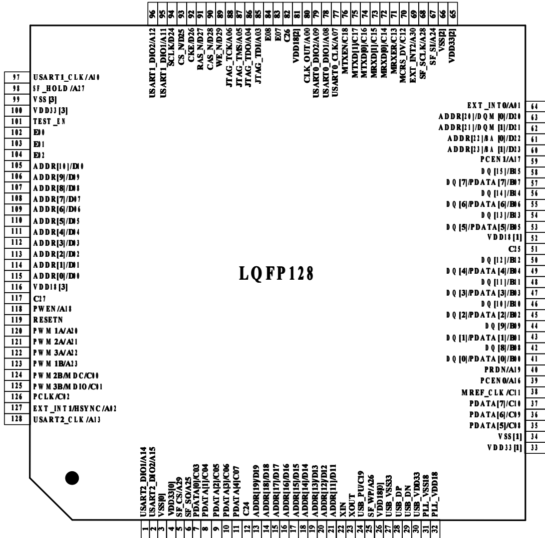
图 3-2 BR8220 引脚分布图
