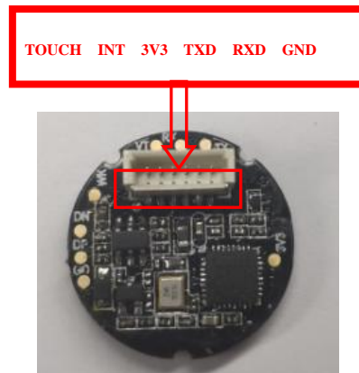
图 3-1 BFM530E 模块图正面
