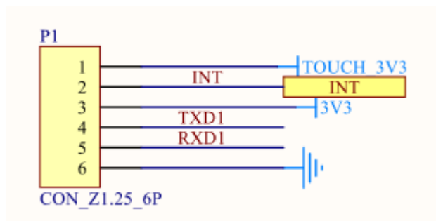
图 3-3 BFM530E 串口接口(P1)
