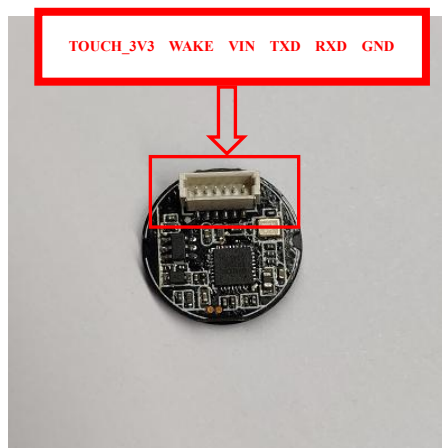
图 3-1 BFM232Y 模块图正面
