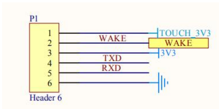
图 3-3 BFM232Y 串口接口(P1)
