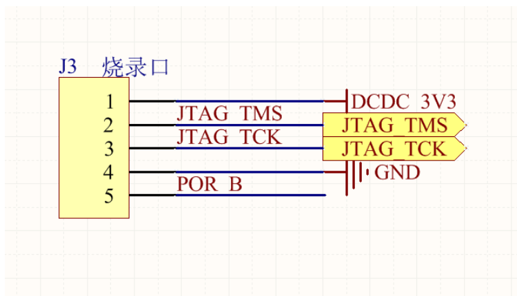
图 3-5 BFC500 烧录接口
