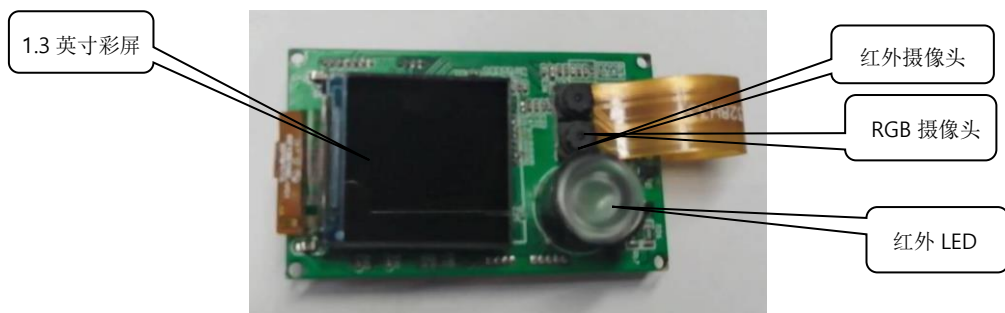
图 3-1 BFC500 模块正面
