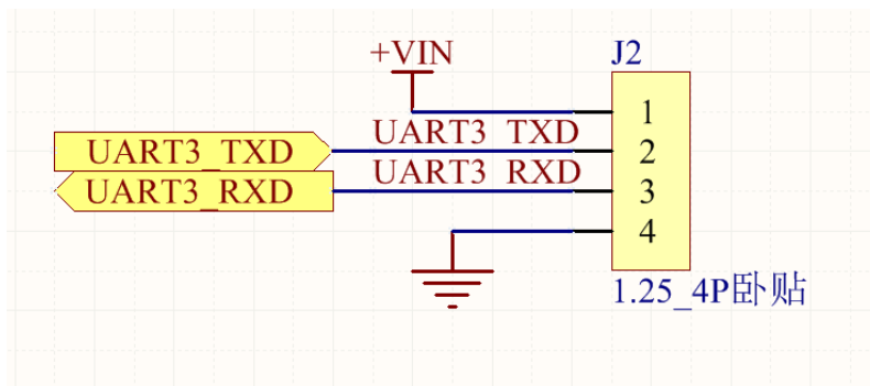
图 3-4 BFC500 UART3 接口
