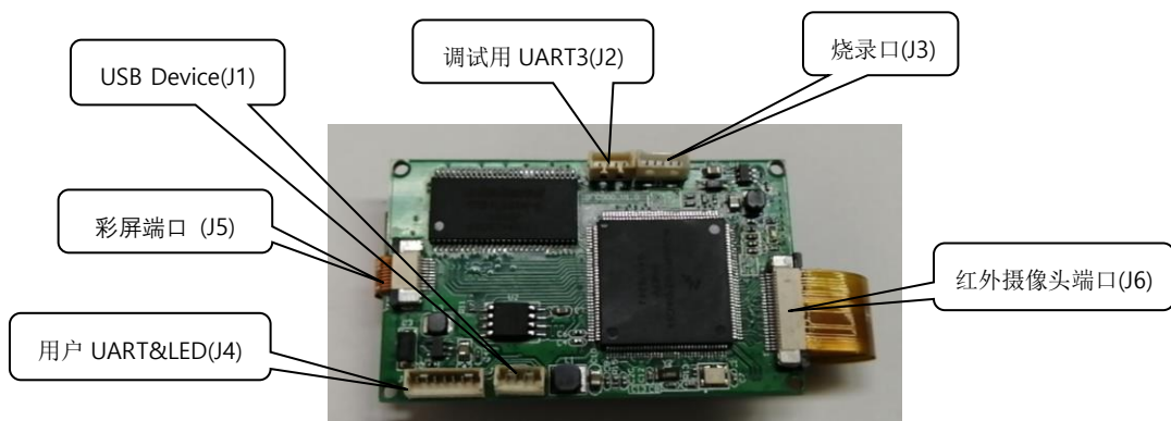
图 3-2 BFC500 模块背面
