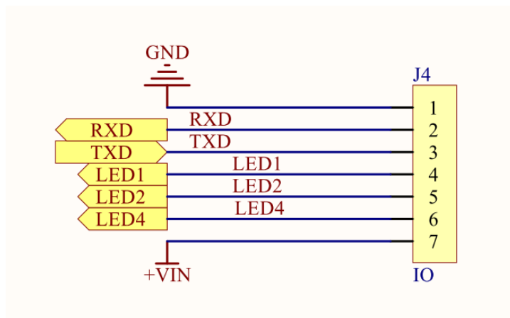
图 3-6 BFC500 用户 UART&LED 接口
